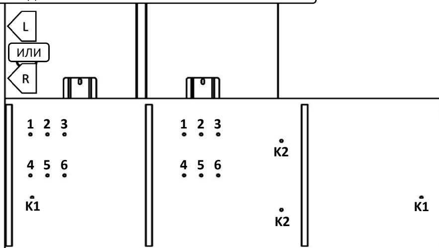
СХЕМА 2.2 - СВЕРЛЕНИЕ ОТВЕРСТИЙ В ВЕРХНЕЙ КРЫШКЕ ТУМБЫ
