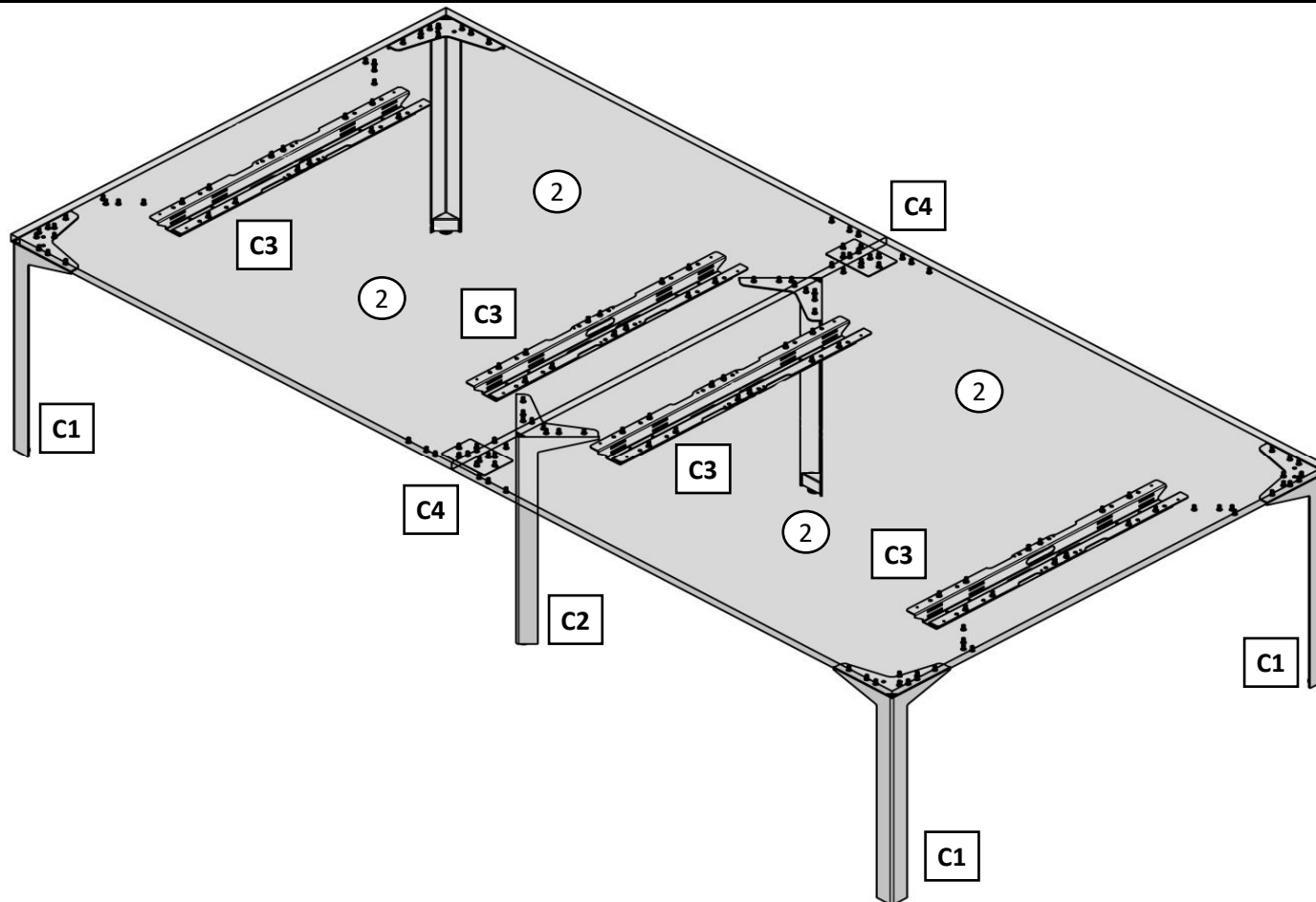
УСТАНОВКА ПЛАСТИНЫ
