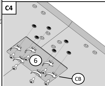
УСТАНОВКА ПЛАСТИНЫ
