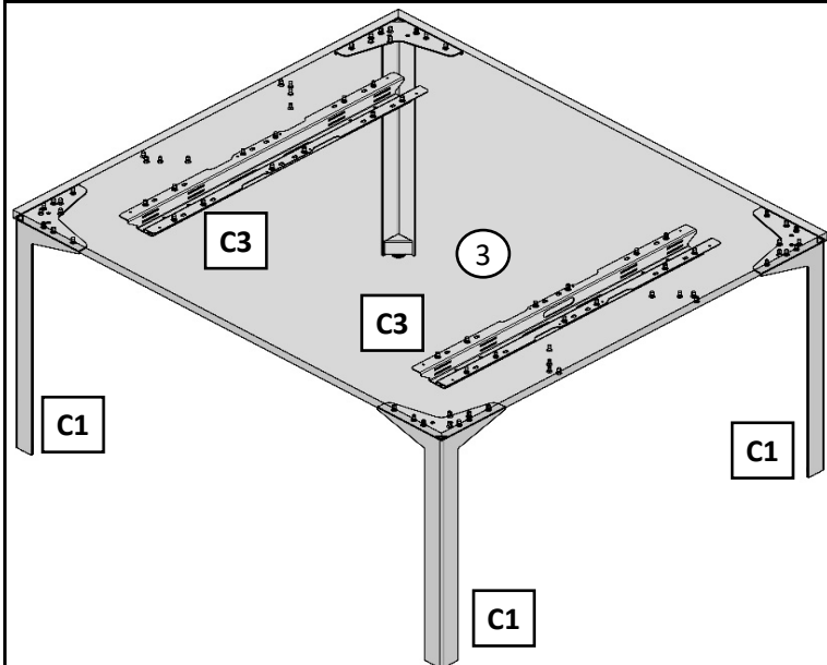
ПЕРЕГОВОРНЫЙ СТОЛ
