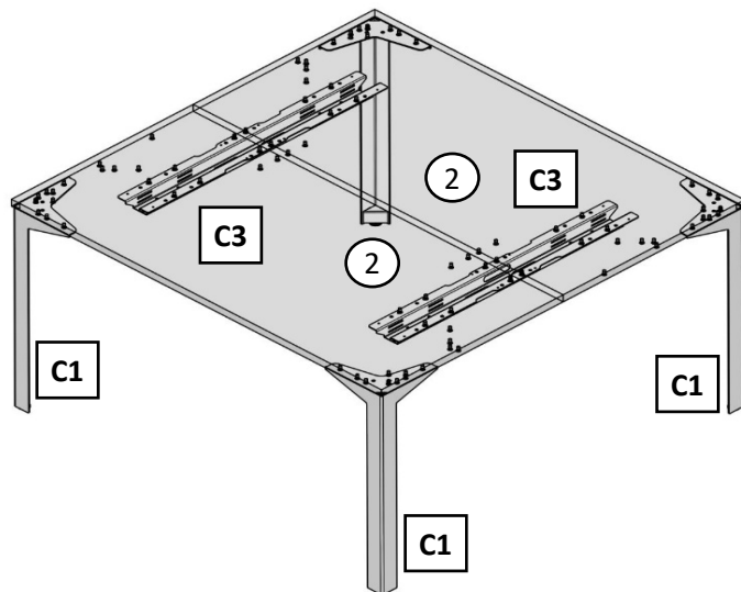
УСТАНОВКА ТРАВЕРСЫ
