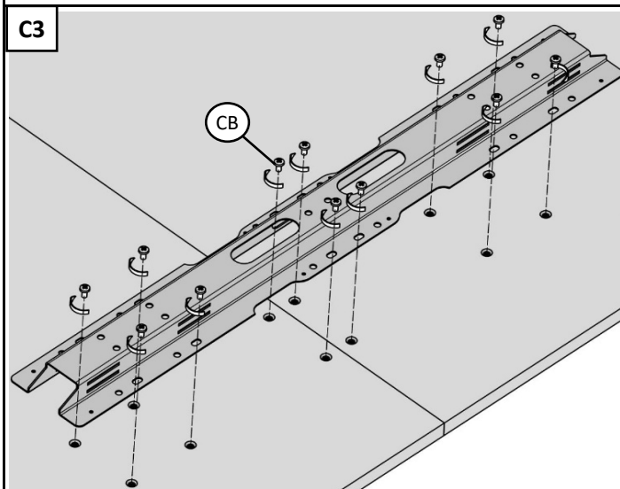
УСТАНОВКА ТРАВЕРСЫ
